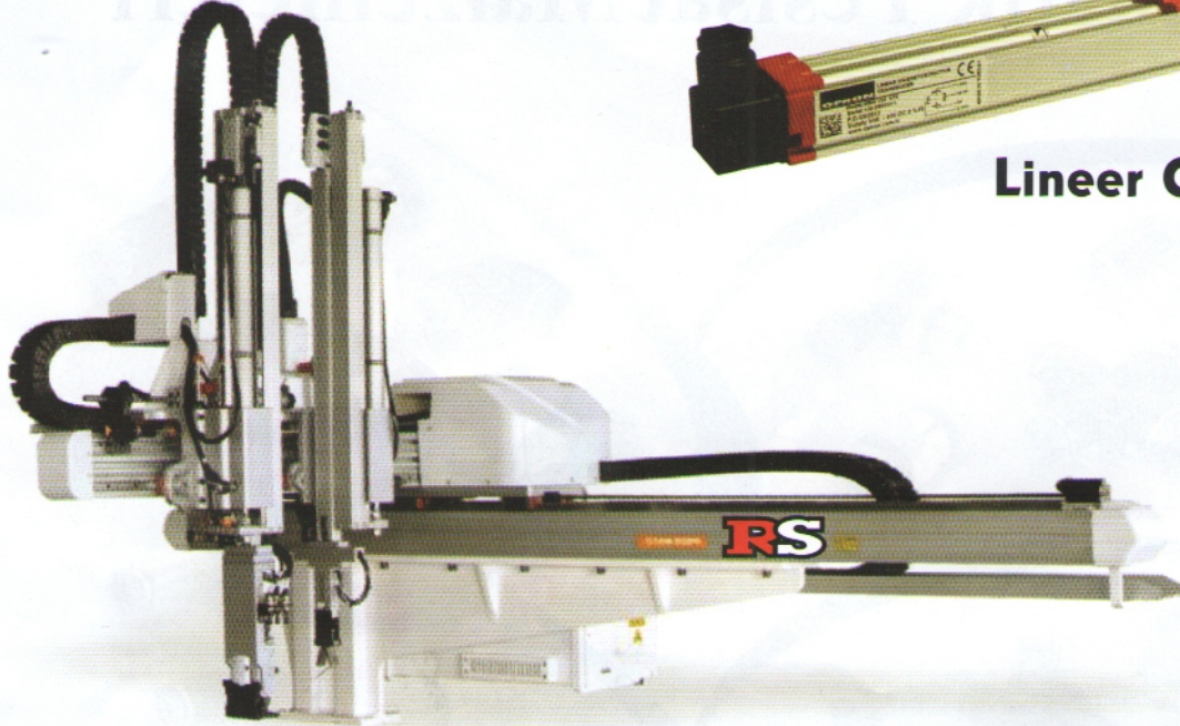
Enjeksiyon Robot Ekipmanları
