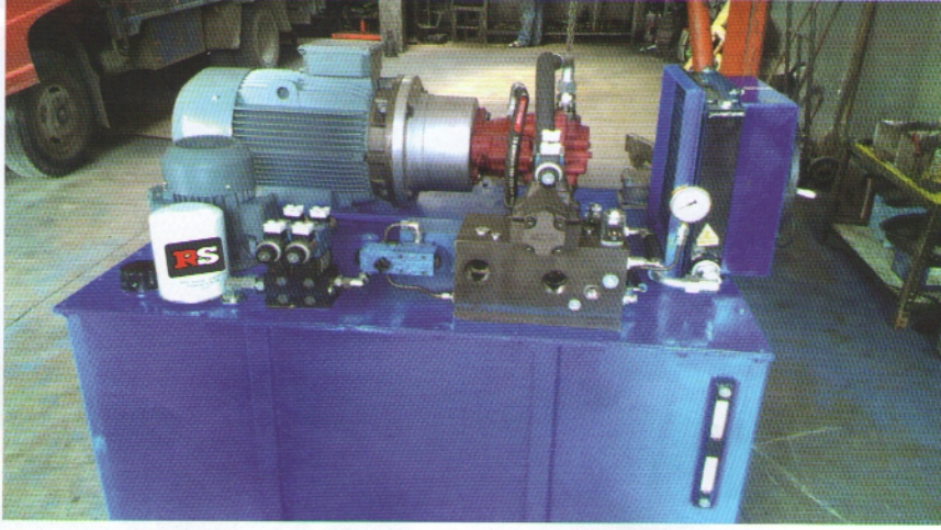
Hidrolik Yağ Ünitesi
